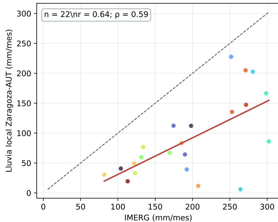
IMERG vs lluvia local
