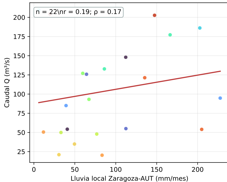
Lluvia local vs caudal
